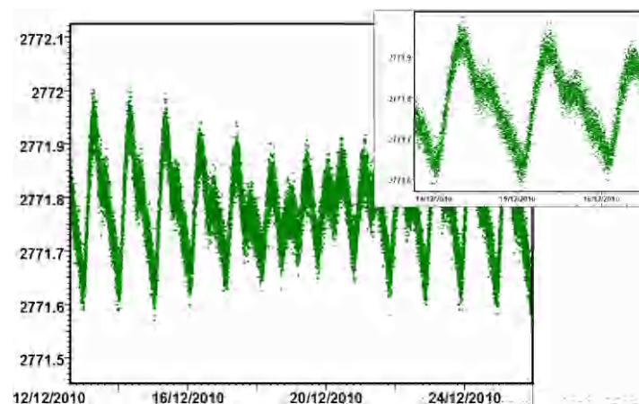
Fig. 11.E.13 – Tides
