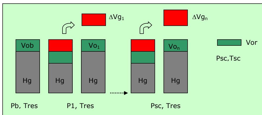
Fig. 9.J.3 – DLE schematic
