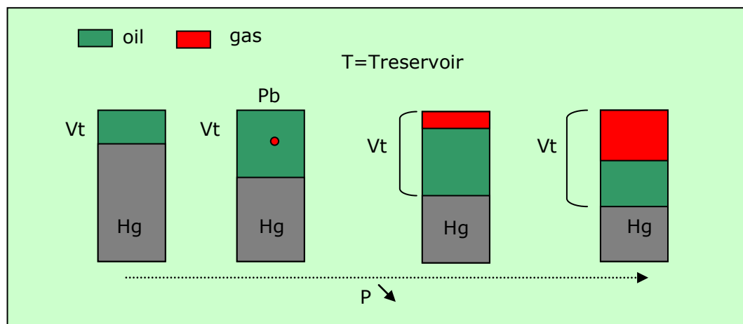
Fig. 9.J.1 – CCE schematic
