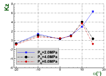
(d) Normal moment amplification factor
