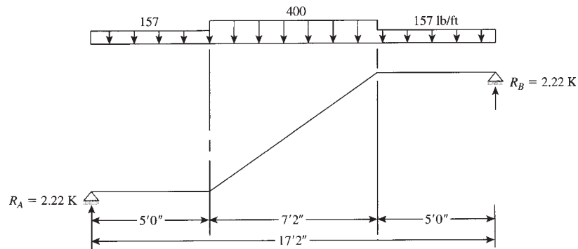
(d) Loads.
