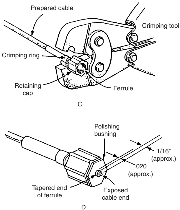
Figure 11-11. (C) Crimping operation. (D) Spacing in ferrule.
