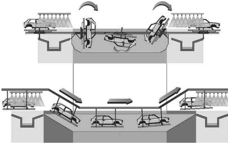
Fig. 3.9 RoDip3 line (source : Dürr).
