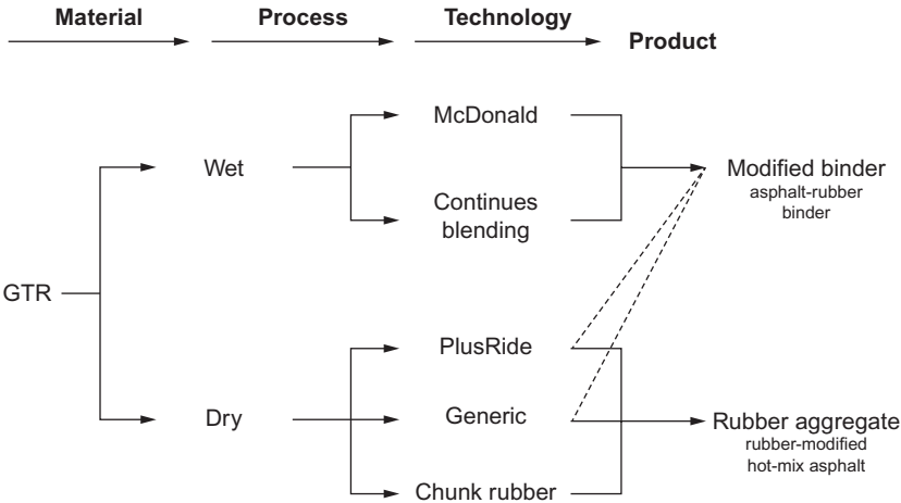
Fig. 6.5 GTR use in HMA.
