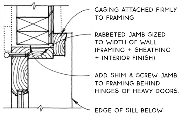
Side Jamb
