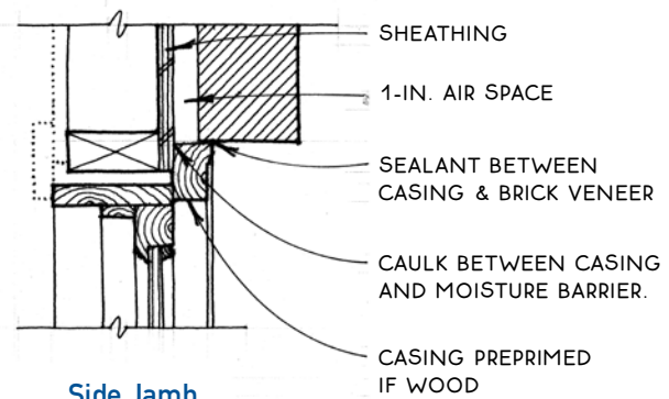
Side Jamb
