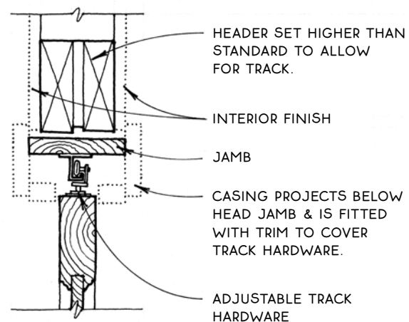
Head Jamb
