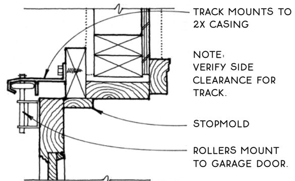
Side Jamb
