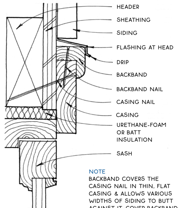
Backband
