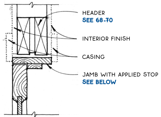
Head Jamb
