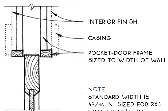
Side Jamb
