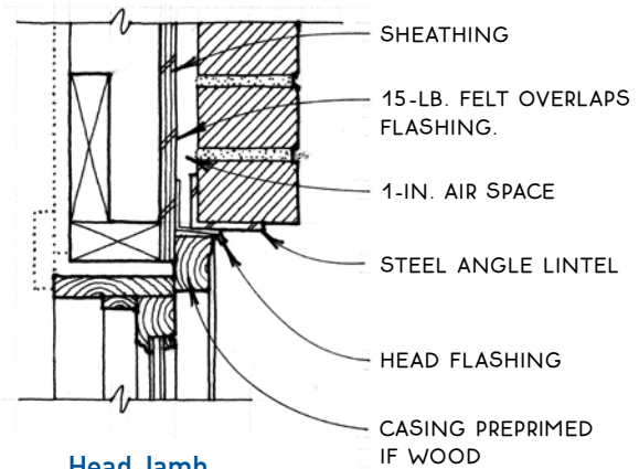
Head Jamb
