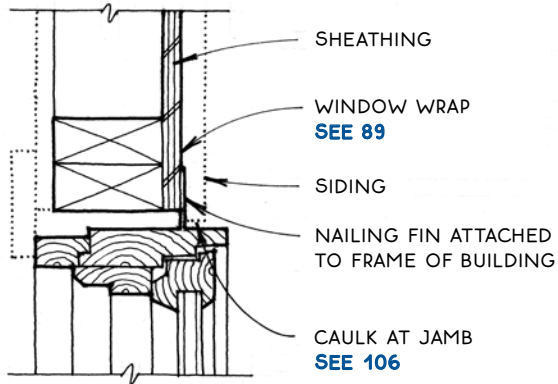
Side Jamb
