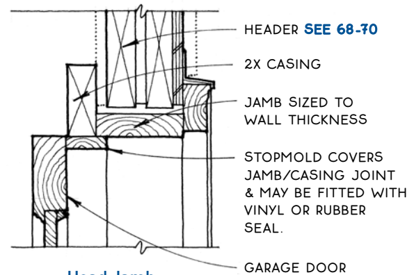
Head Jamb
