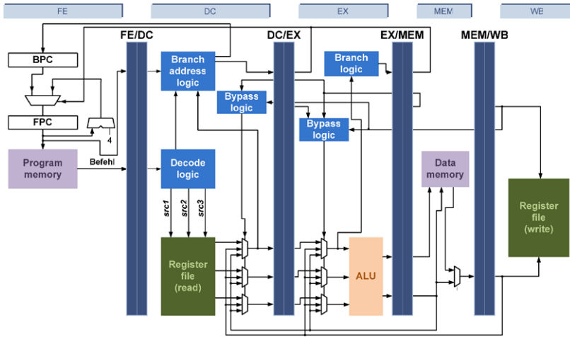
Fig. 2.19 ASIP-template (LT_RISC).
