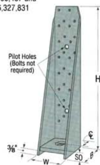
HHDQ11 (HHDQ14 similar)
