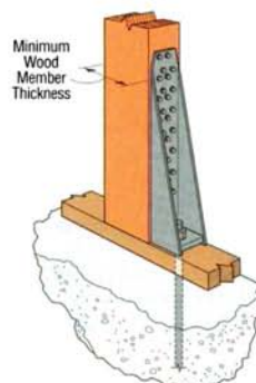
Vertical HHDQ11 Installation (HHDQ14 similar)
