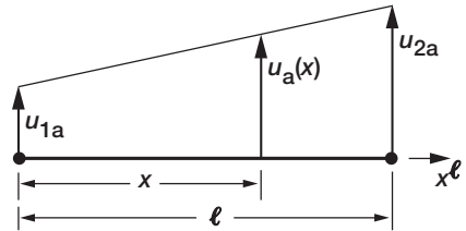
(d) Linear displacement function.
