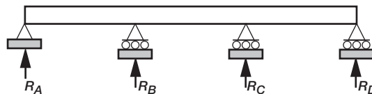
(d) Force model 3.
