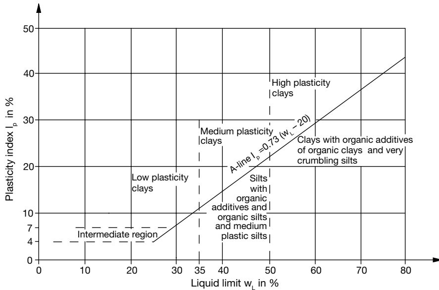
Figure 2.16 Plasticity (Casagrande) chart. (After DIN 2006.)
