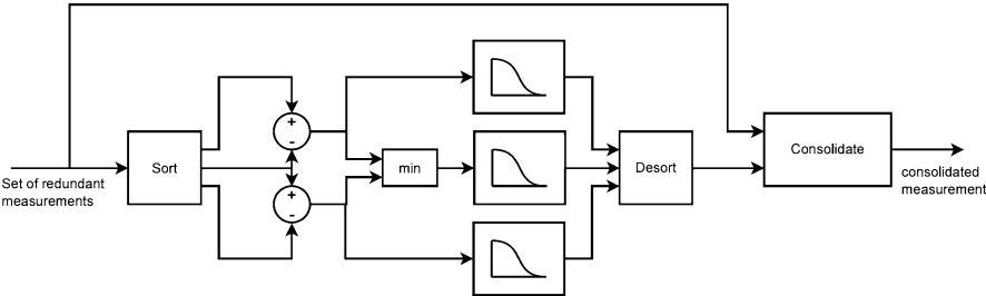
Fig. 5.7 Soft voter
