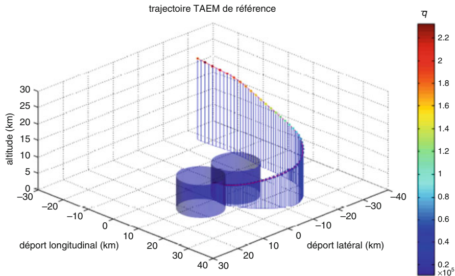
Fig. 7.31 TAEM trajectory
