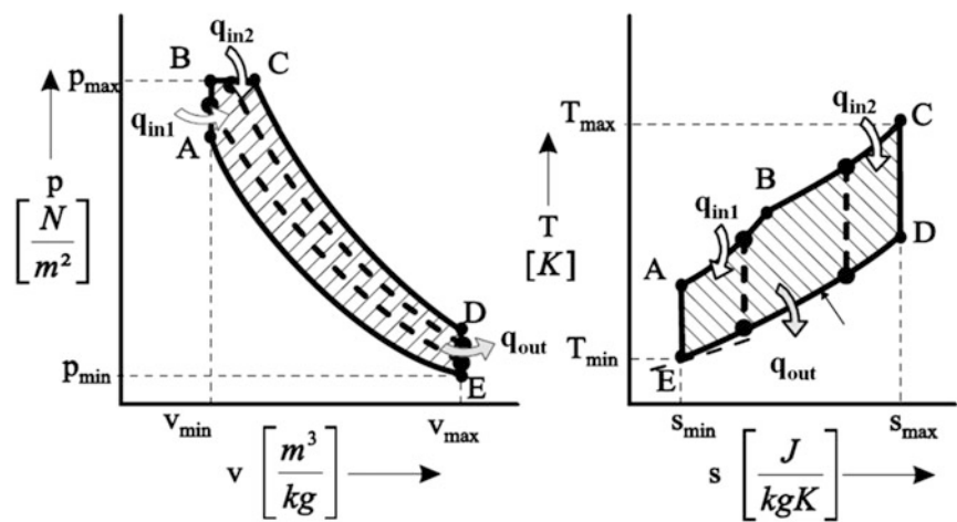
Fig. 2.5 Seiliger cycle
