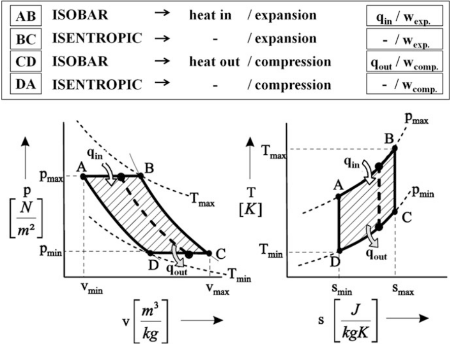
Fig. 2.6 Joule cycle
