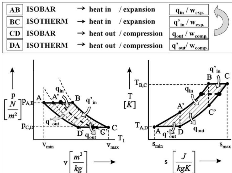
Fig. 2.7 Ackeret-Keller cycle
