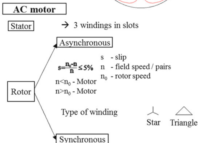
Fig. 4.6 AC motor
