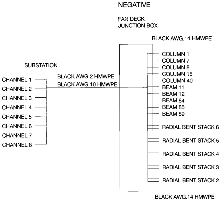
Fig. 3.6 Fan deck junction box.
