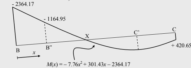
b1) Bending moment diagram
