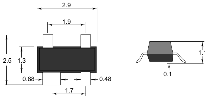
Fig. 2.88 SOT-143 package
