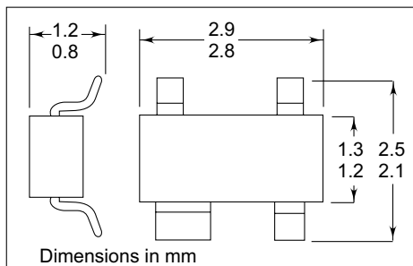
Fig. 2.85 SOT-23 package
