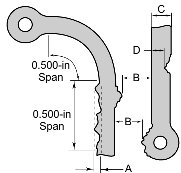
Fig. 14.21 Edge definition
