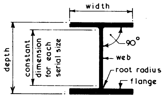
UNIVERSAL COLUMNS
