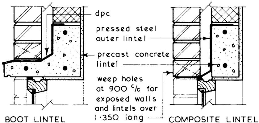
BOOT LINTEL
