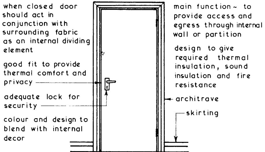
INTERNAL DOOR
