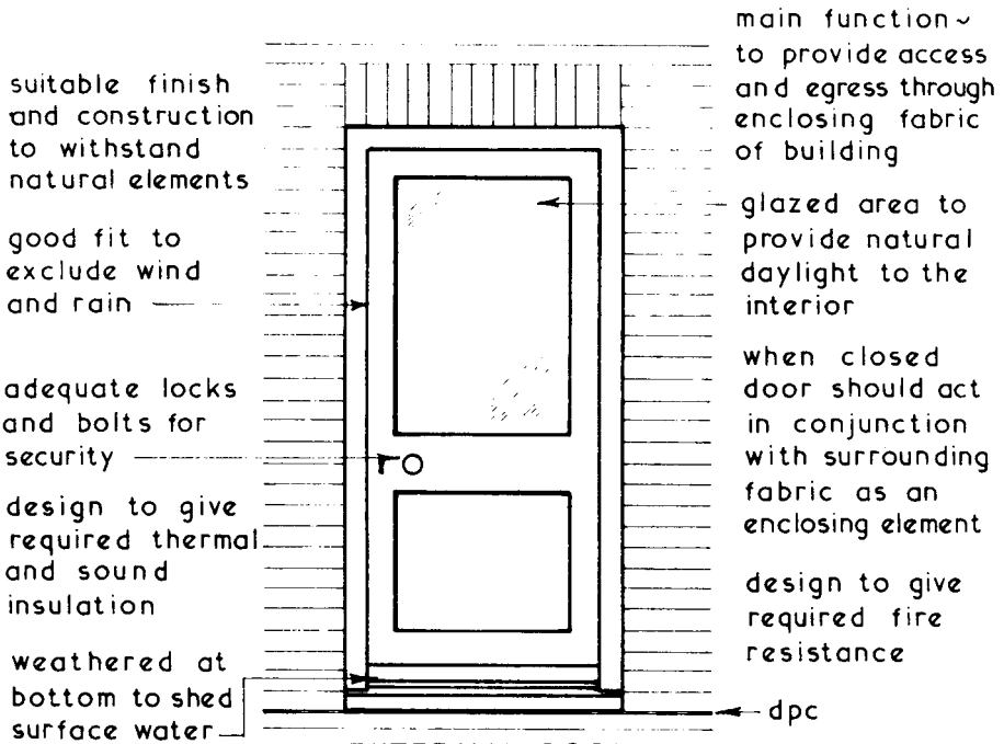
EXTERNAL DOOR
