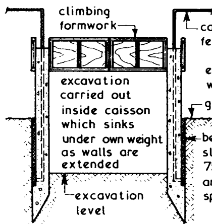
LAND CAISSON
