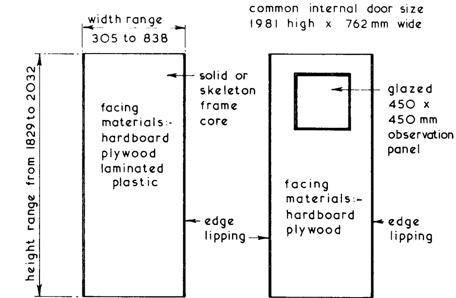
FLUSH DOOR
