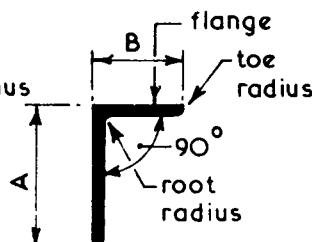
UNEQUAL ANGLES
