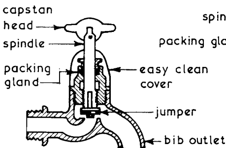
BIB TAP
