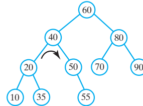
(d) After right rotation about 40
