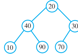
(d) After reheap(2)
