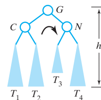
(d) After right rotation
