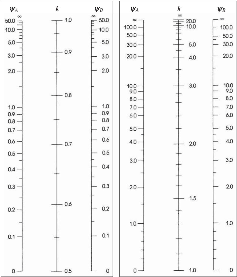
Nonsway frames Sway frames
