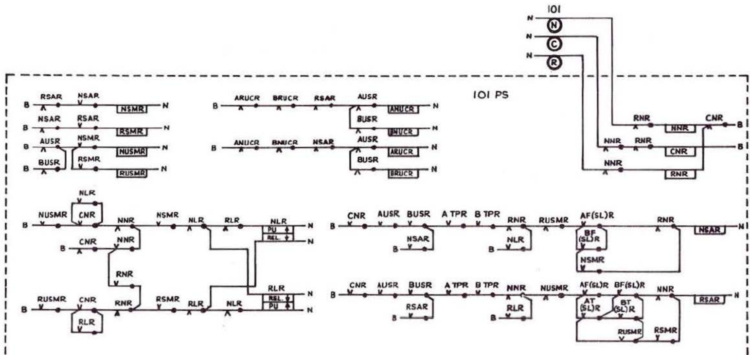
Fig. 6:9 System A: point setting circuit
