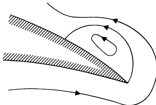
Fig. 8.12. The starting vortex.
