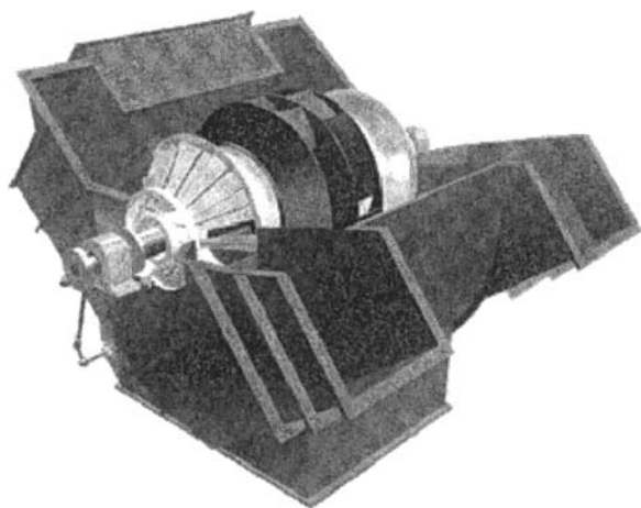
Figure 3.4 Centrifugal fan
