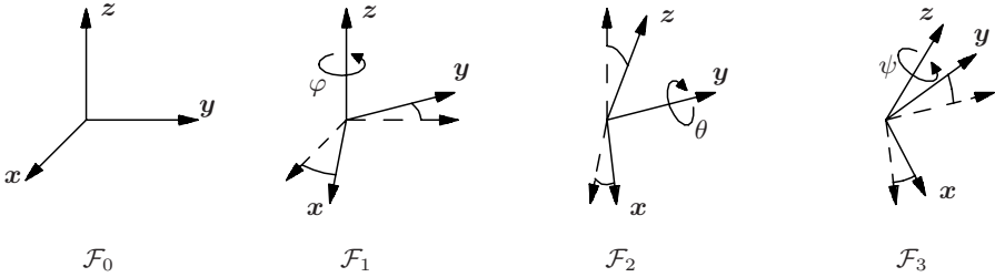
Fig. C.3. Euler angles.
