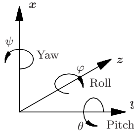
Fig. C.4. RPY angles.
