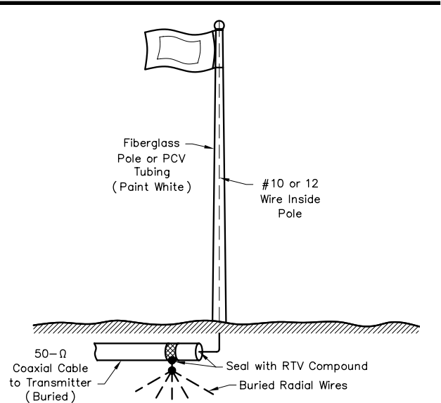
Fig 6—A flagpole antenna.
