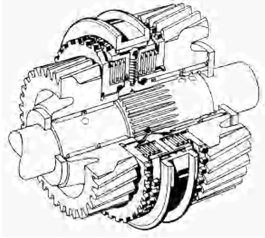
Fig. 9.28. Multi-plate synchronizer
