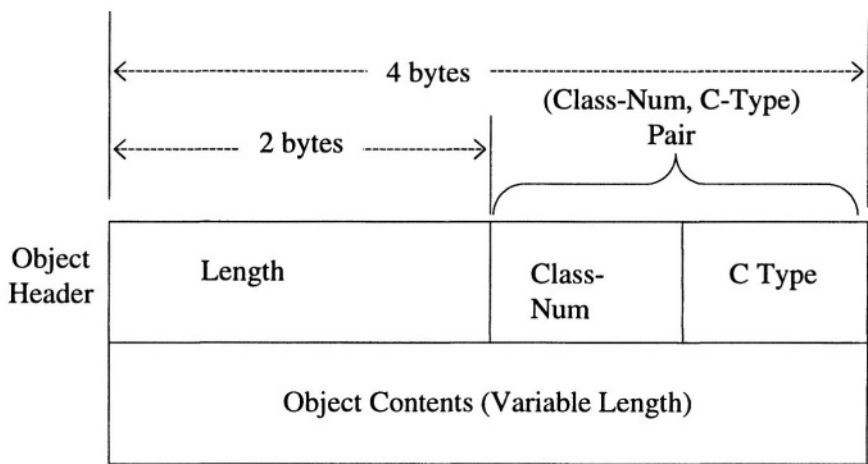
Figure 5-6. RSVP message object format.
