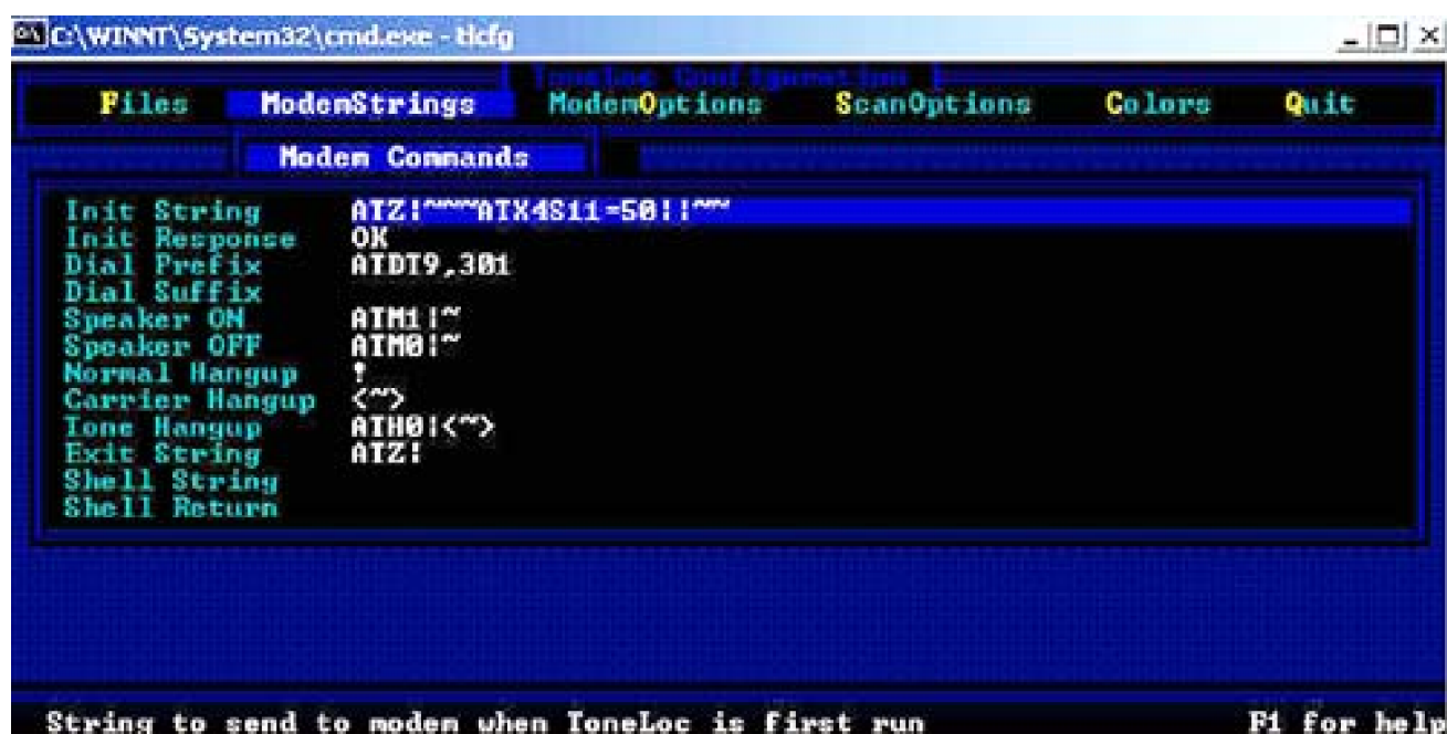
Figure 6-3. ToneLoc ModemStrings menu
