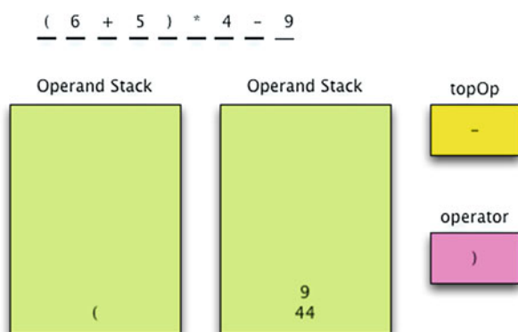
Fig.4.17 Infix Evaluation Step 3
