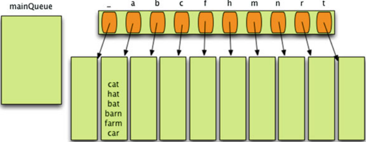
Fig.4.23 Radix Sort Step 6—2nd letter
