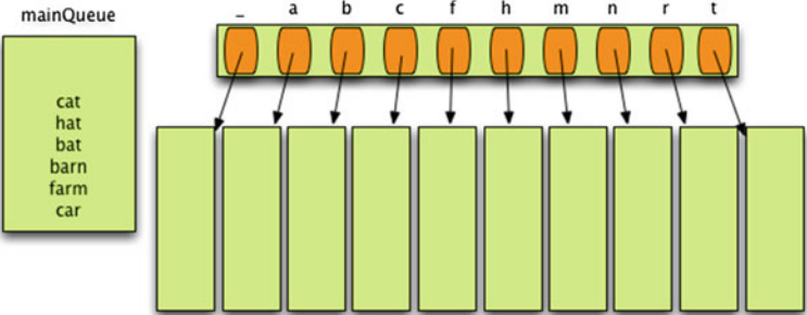
Fig.4.24 Radix Sort Step 7
