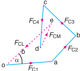
(f) Force polygon.
