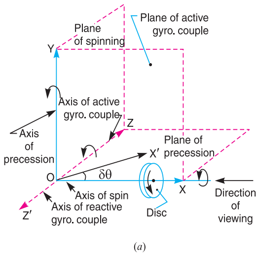
Fig. 14.2. Gyroscopic couple.
