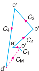
(e) Couple polygon.
