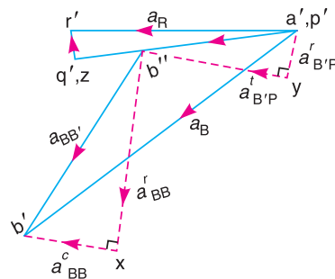
(d) Acceleration diagram.
