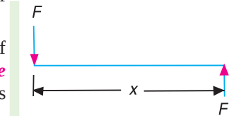
Fig. 3.2. Couple.
