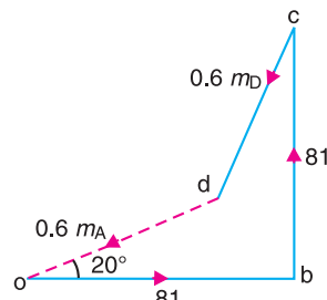
(d) Force polygon.
