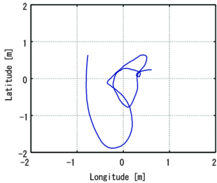
Fig. 5.37 Hovering result of SF40
