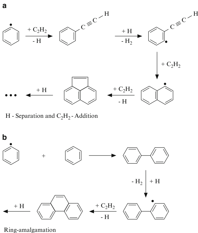
Fig. 6.18 PAH growth, acc. to nach Frenklach and Wang (1994)
