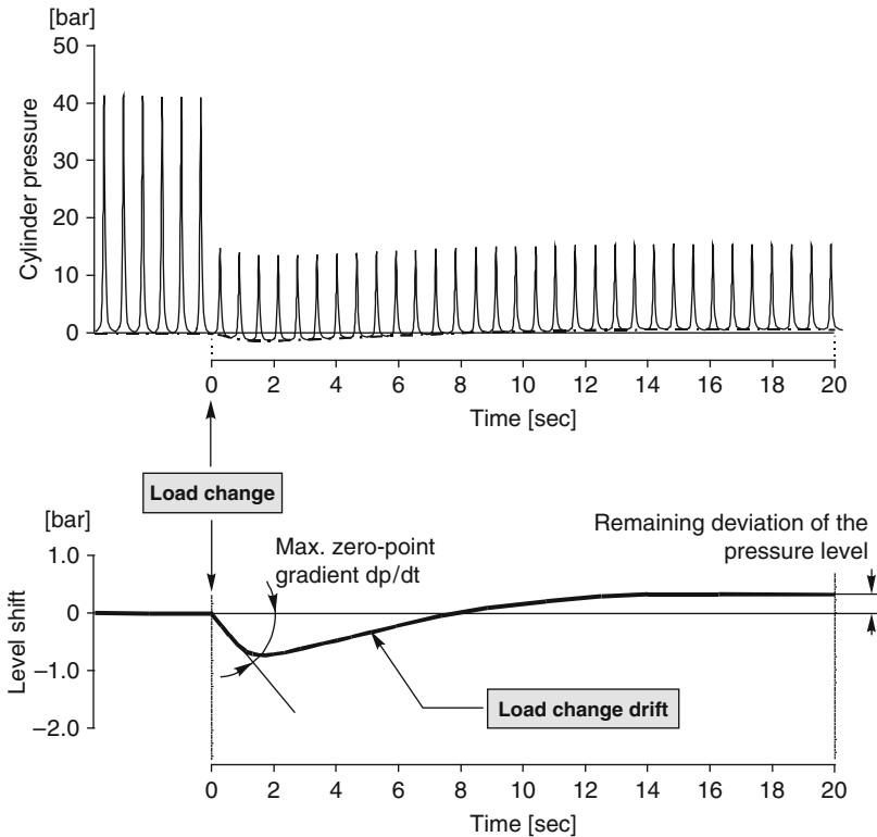
Fig. 3.15 Load change drift
