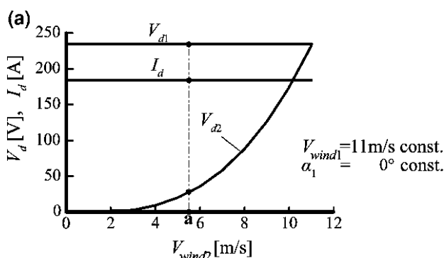
I_d , V_{d1} , V_{d2} versus V_{wind2} .
