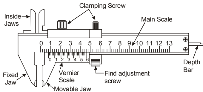
Fig. Vernier calliper
