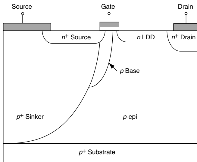
(B) Lateral MOSFET
